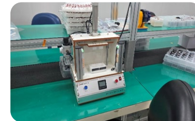
소형 프레스 설비 안전커버 설치
